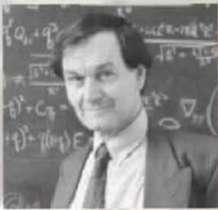
Roger Penrose
