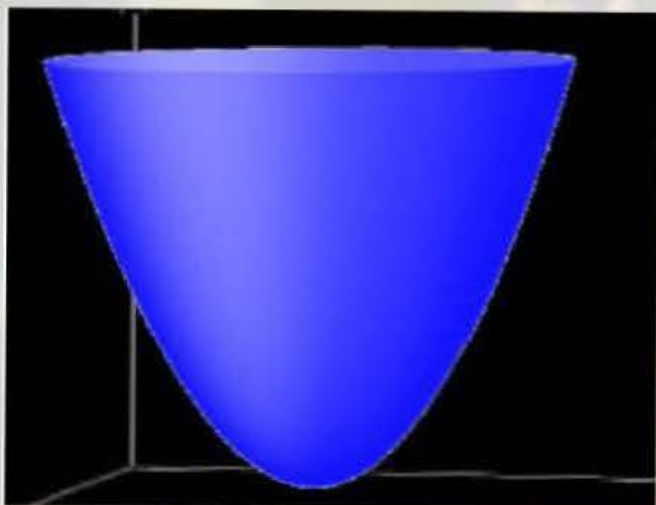
En el modelo cosmológico de Hartle-Hawking, el espacio-tiempo no comienza en un vértice afilado, sino en un extremo redondeado. Así pues, no hay singularidad inicial.
