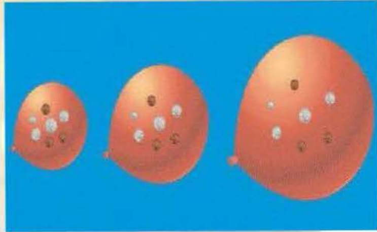
La expansión cosmológica equivale a la separación de las monedas pegadas sobre un globo que se infla. No se mueven las monedas; su distancia mutua aumenta al estirarse la goma sobre la que están pegadas.
